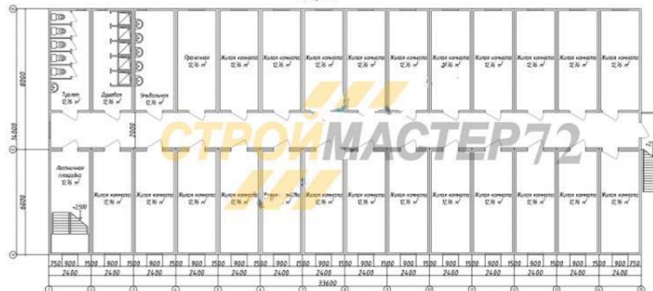
Модульное общежитие из 56 БК 2 этаж 470,4 м 2
